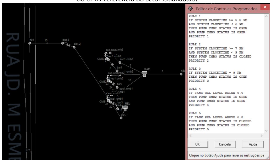
Figura 113: controles programados aplicados para determinação da rotina operacional do SAA referência do setor Guanabara.
