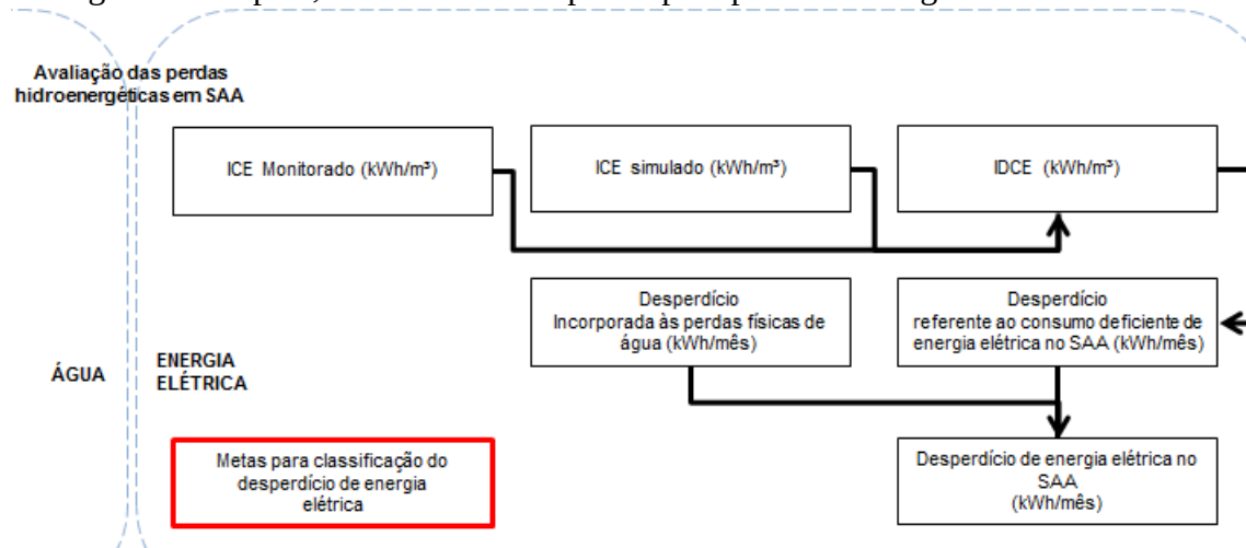
Figura 46: etapa 4, classes de desempenho para perda de energia elétrica no SAA.
