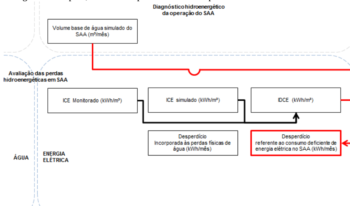
Figura 44: etapa 4, calculo das perdas de elétrica por excesso no consumo no SAA.
