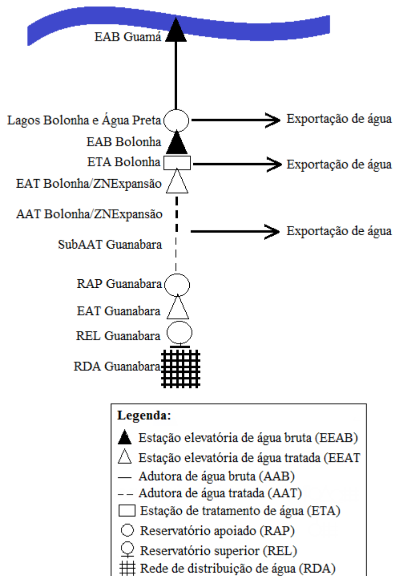
Figura 115: linha hidroenergética do SAA Guamá/Bolonha/Zona de expansão/Guanabara.
