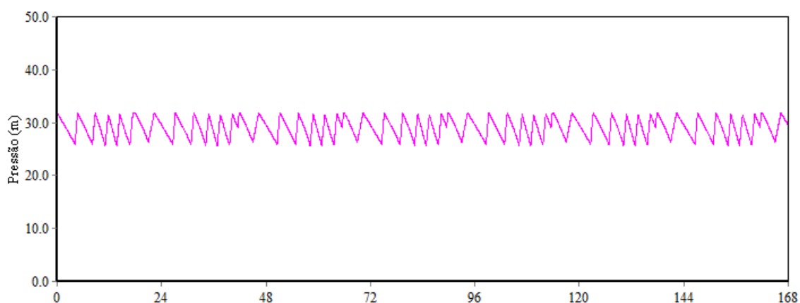
Gráfico 44: pressão no ponto mais desfavorável da RDA do SAA referência.
