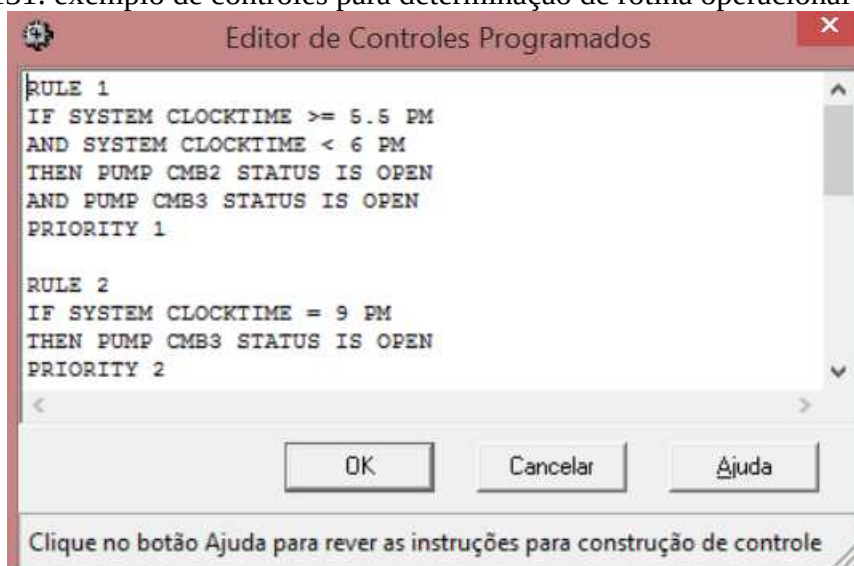
Figura 131: exemplo de controles para determinação de rotina operacional em SAA.
