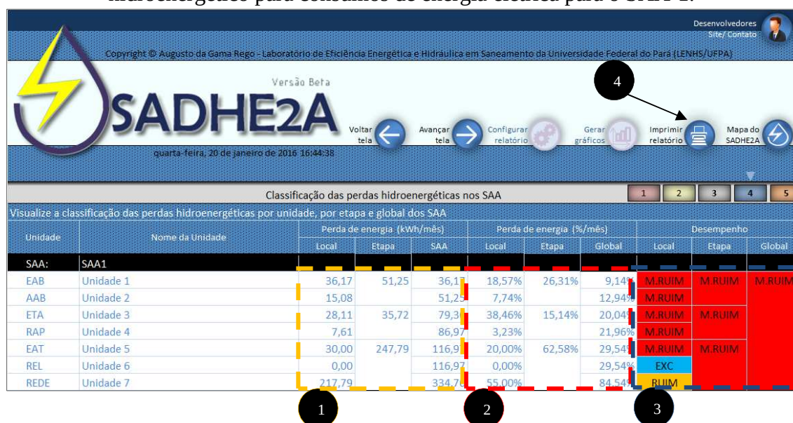
Figura 170: SADHE2A – avalia – Dashboard com avaliação do desempenho hidroenergético para consumos de energia elétrica para o SAA-1.
