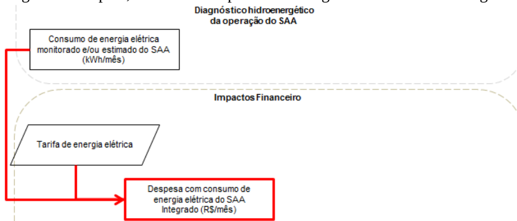
Figura 50: etapa 5, cálculo da despesa com energia elétrica no SAA integrado.
