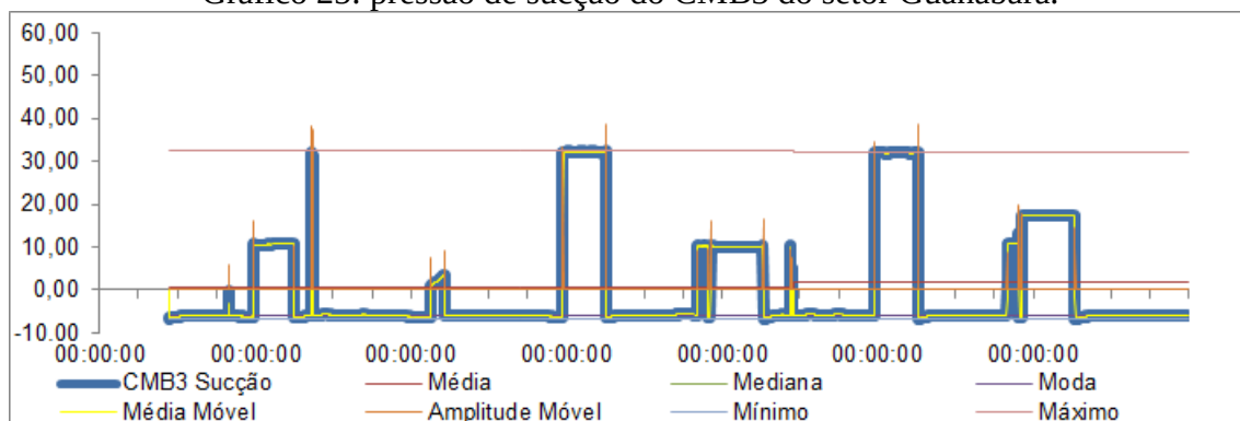
Gráfico 25: pressão de sucção do CMB3 do setor Guanabara.
