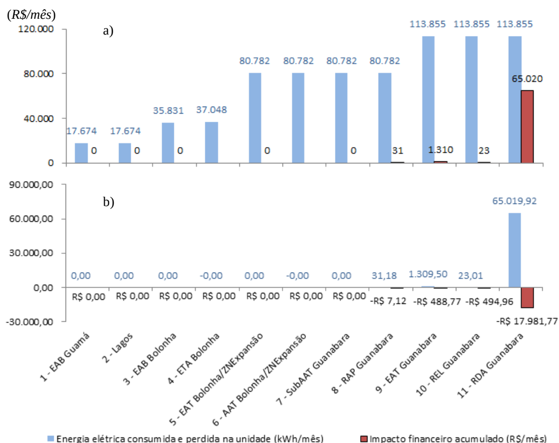
Gráfico 54: energia elétrica diagnosticada base total (Eb T,d,i ) e acumulada e energia elétrica diagnosticada base perdida (Eb p,d,i ) no SAA Guanabara. b) energia elétrica diagnosticada base perdida (Eb p,d,i ) e o impacto financeiro acumulado (IFbT i ) no SAA Guanabara.
