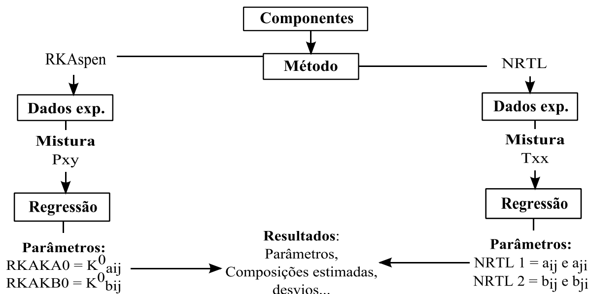
Figura 1.7 – Ajuste de parâmetros no Aspen Properties®.
