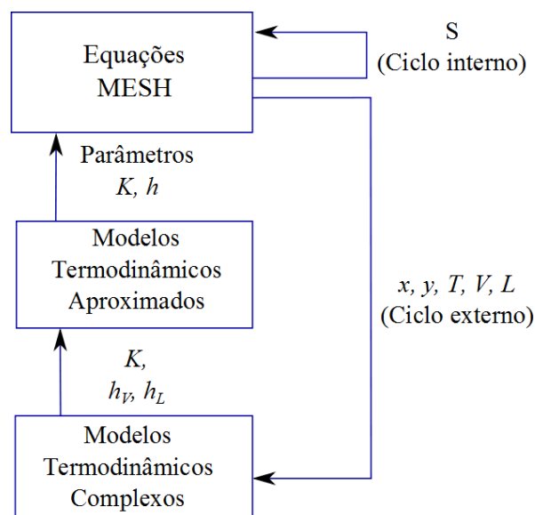
Figura 1.6 – Incorporação de correlações de propriedades termodinâmicas em ciclos iterativos (método inside-out ).
