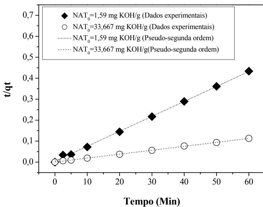
Figura D. 4 - Modelo cinético de pseudo-segunda ordem da adsorção de ácidos graxos livres em lama vermelha ativada termicamente a 400°C.
