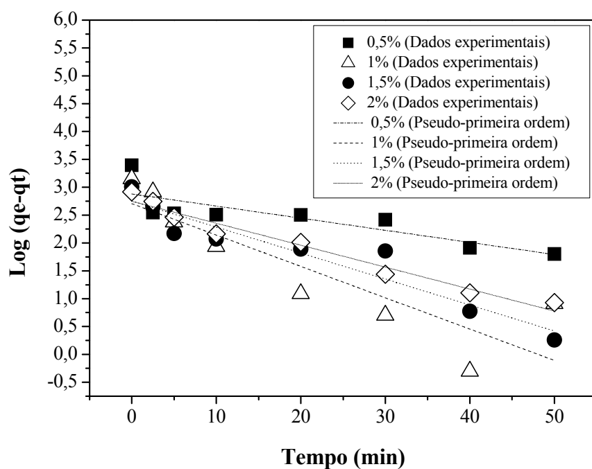
Figura D. 7 - Modelo cinético de pseudo-primeira ordem da adsorção de ácidos graxos livres em lama vermelha ativada quimicamente com 0,25M HCl.
