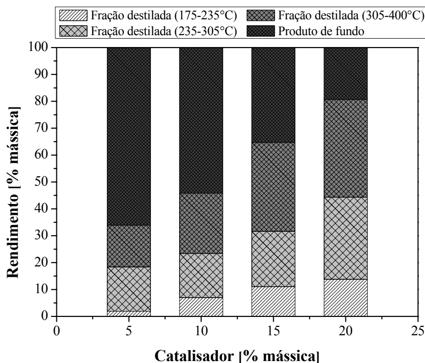
Figura 4. 4 – Efeito da porcentagem de catalisador sobre o rendimento das frações destiladas a partir do PLO.
