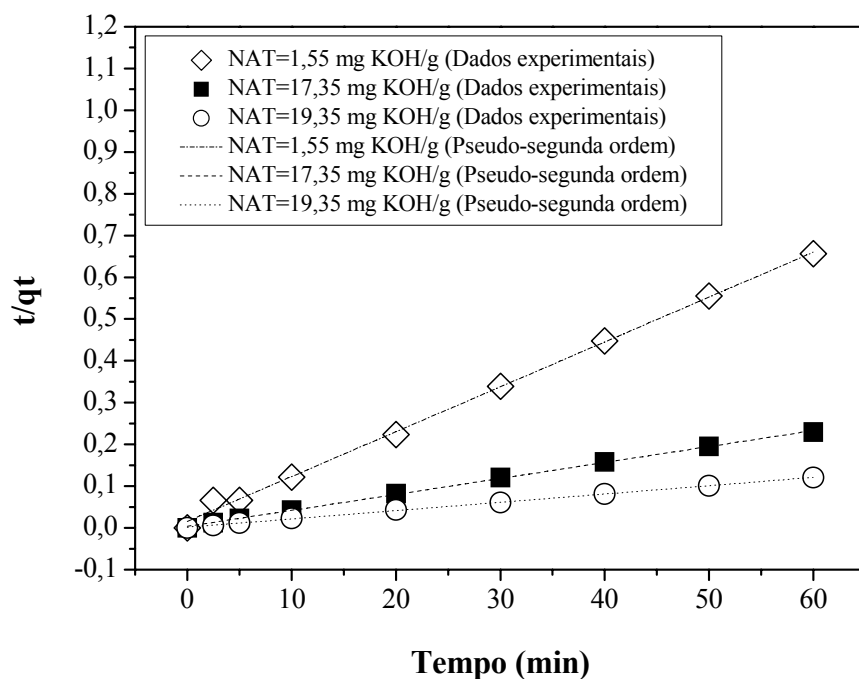
Figura D. 2 - Modelo cinético de pseudo-segunda ordem da adsorção de ácidos graxos livres em em alumina ativada a 450°C.
