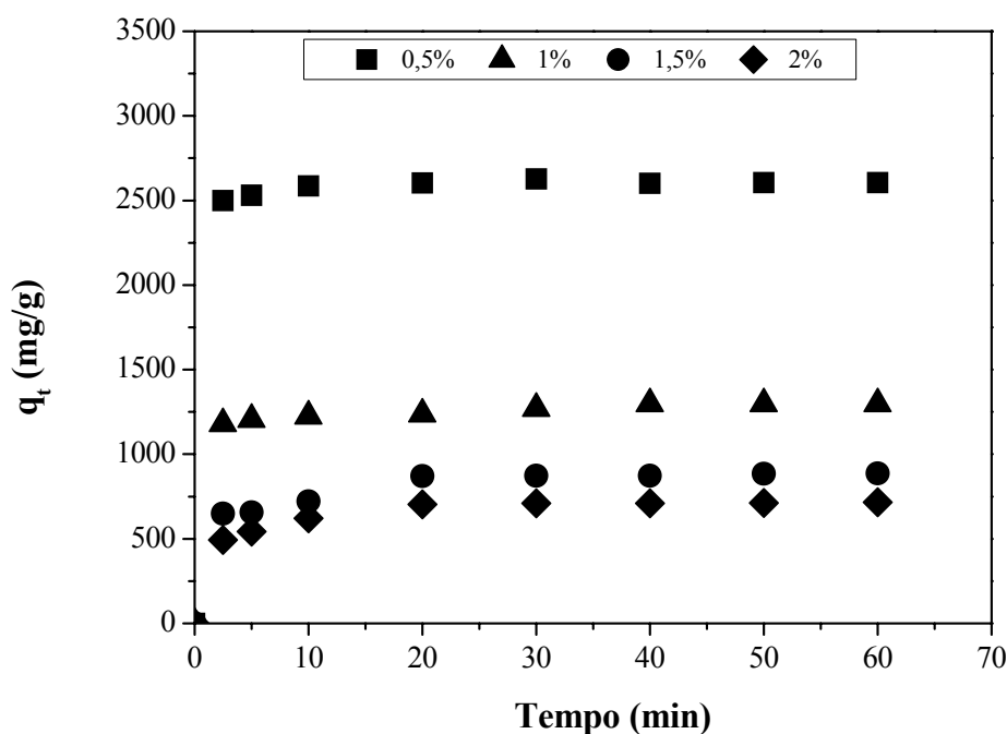
Figura 6. 17 – Cinética de adsorção de AGL a partir de fração destilada na faixa da gasolina com lama vermelha ativada quimicamente com 2M HCl como adsorvente: efeito da porcentagem de adsorvente.
