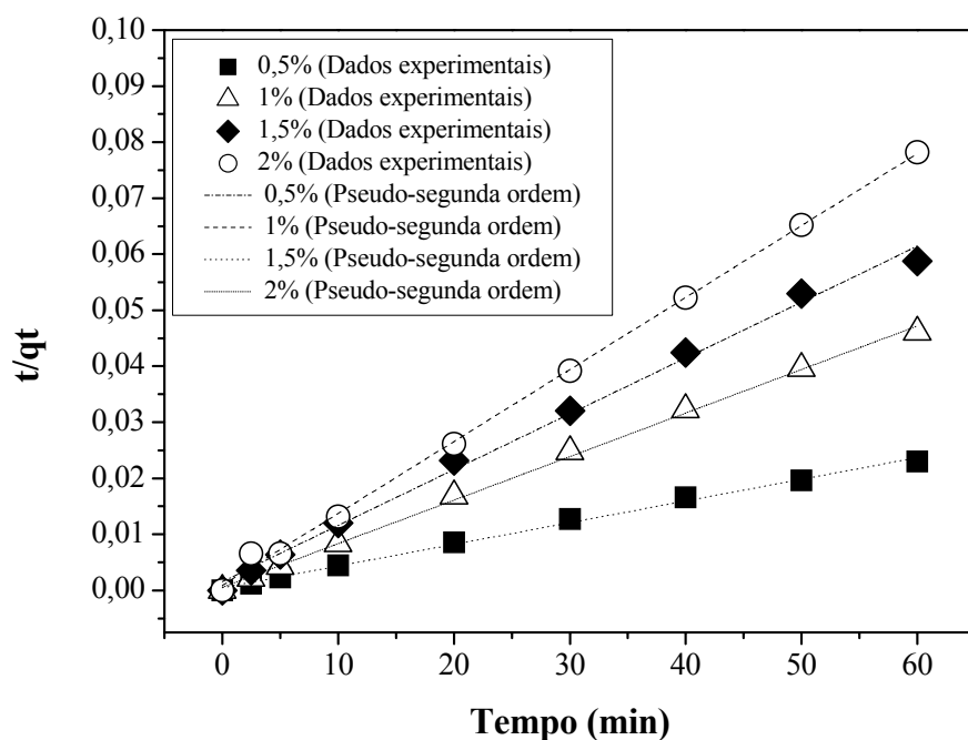
Figura D. 8 - Modelo cinético de pseudo-segunda ordem da adsorção de ácidos graxos livres em lama vermelha ativada quimicamente com 0,25M HCl.
