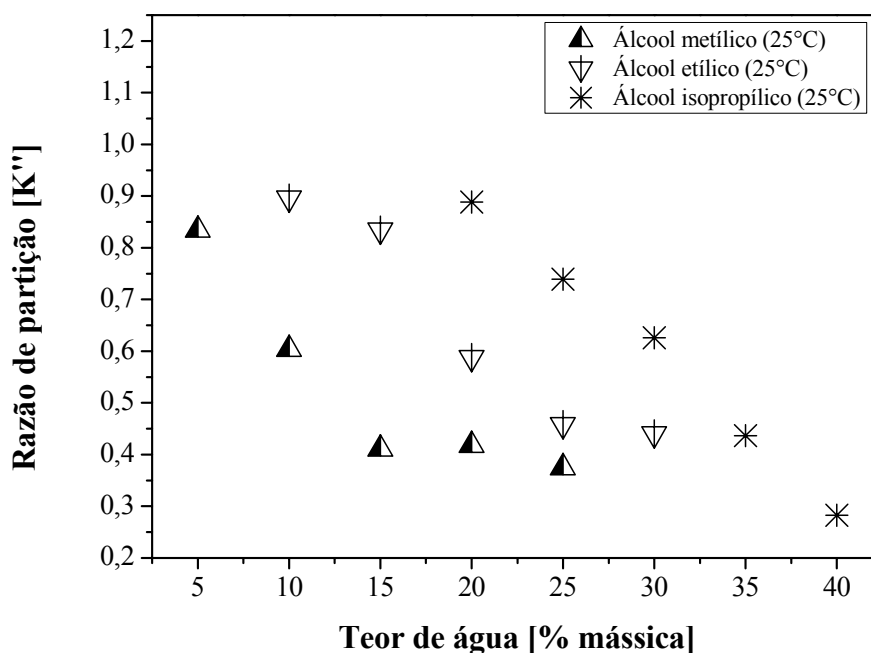
Figura 5. 11 – Razão de partição versus teor de água para diferentes solventes a 25°C.
