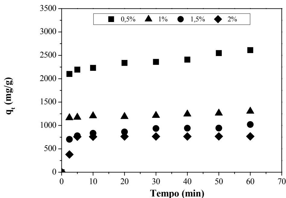
Figura 6. 15 – Cinética de adsorção de AGL a partir de fração destilada na faixa da gasolina com lama vermelha ativada quimicamente com 0,25M HCl como adsorvente: efeito da porcentagem de adsorvente.
