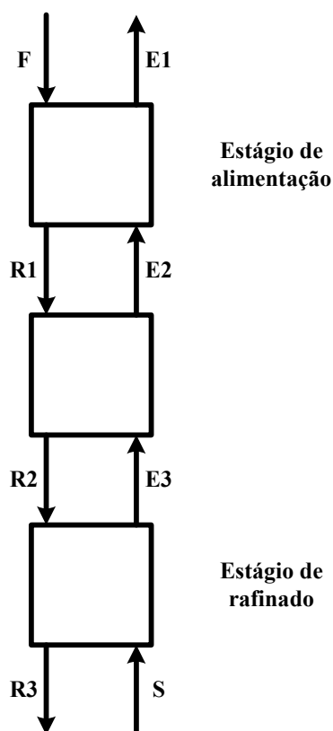
Figura 5. 2 – Extração padrão em contracorrente.
