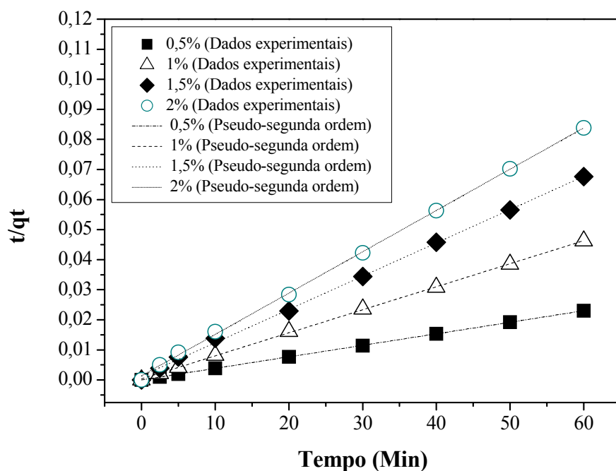
Figura D. 12 - Modelo cinético de pseudo-segunda ordem da adsorção de ácidos graxos livres em lama vermelha ativada quimicamente com 2M HCl.
