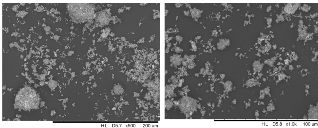
Figura 6. 9 – Microscopia eletrônica de varredura para a lama vermelha ativada termicamente a 600°C.
