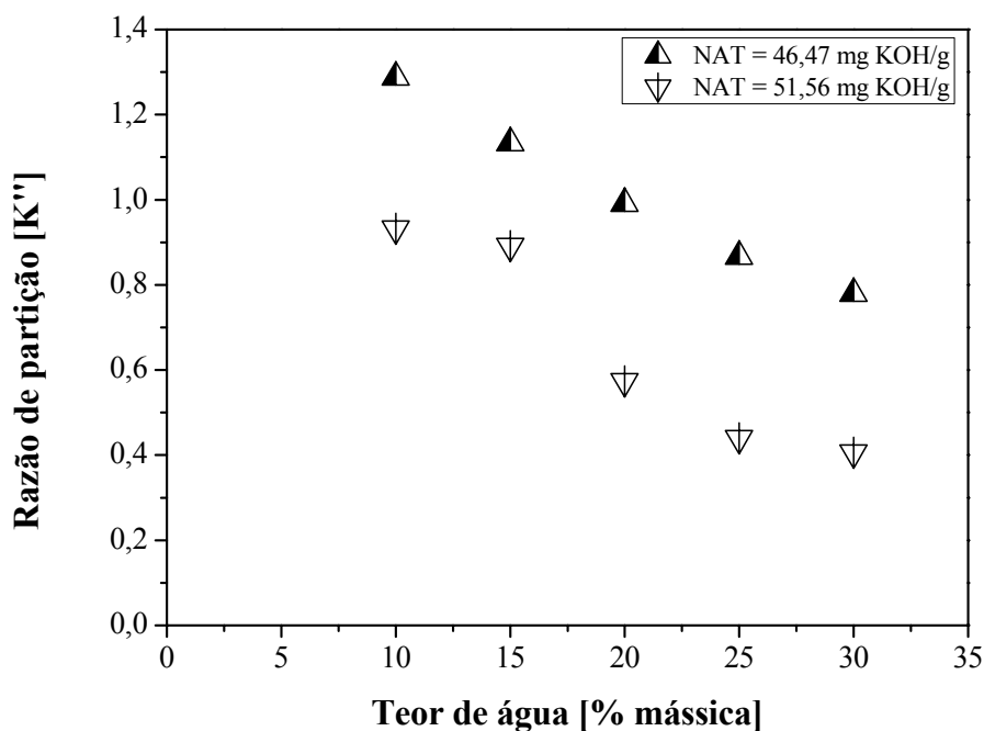
Figura 5. 7 – Razão de partição em função do teor de água (álcool etílico + água).
