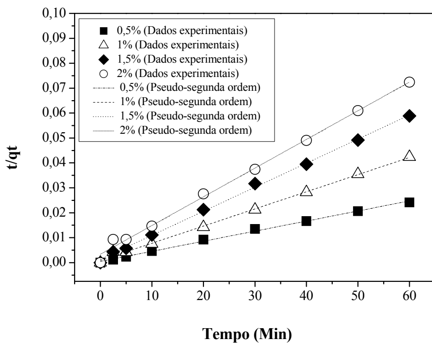
Figura D. 10 - Modelo cinético de pseudo-segunda ordem da adsorção de ácidos graxos livres em lama vermelha ativada quimicamente com 1M HCl.
