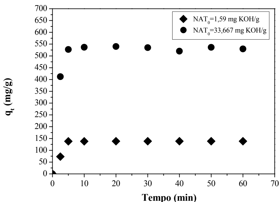
Figura 6. 13 – Cinética de adsorção de AGL a partir de fração destilada na faixa de diesel leve com lama vermelha ativada termicamente a 400°C como adsorvente: efeito da concentração inicial de AGL.
