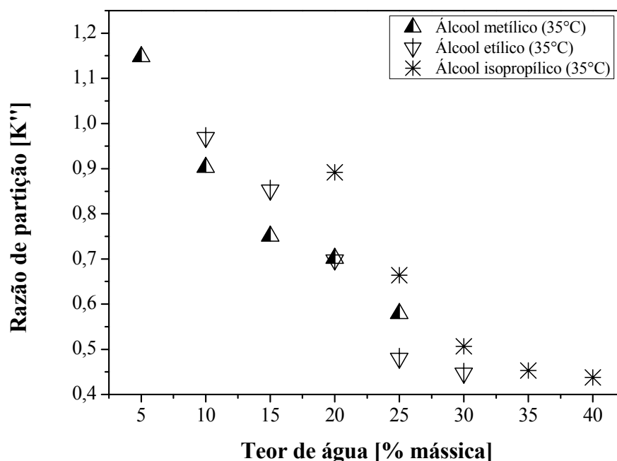
Figura 5. 12 – Razão de partição versus teor de água para diferentes solventes a 35°C.
