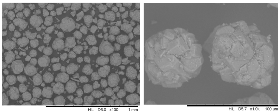
Figura 6. 6 – Microscopia eletrônica de varredura para alumina ativada a 450°C.
