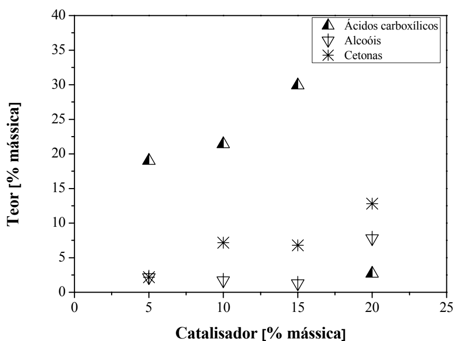
Figura 4. 8 – Distribuição de compostos oxigenados presentes nas frações destiladas (diesel pesado) versus a porcentagem de catalisador empregada no processo de craqueamento.
