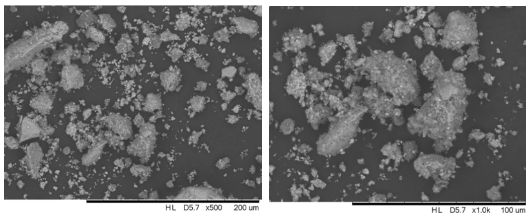
Figura 6. 10 – Microscopia eletrônica de varredura para a lama vermelha ativada quimicamente com 0,25M HCl.
