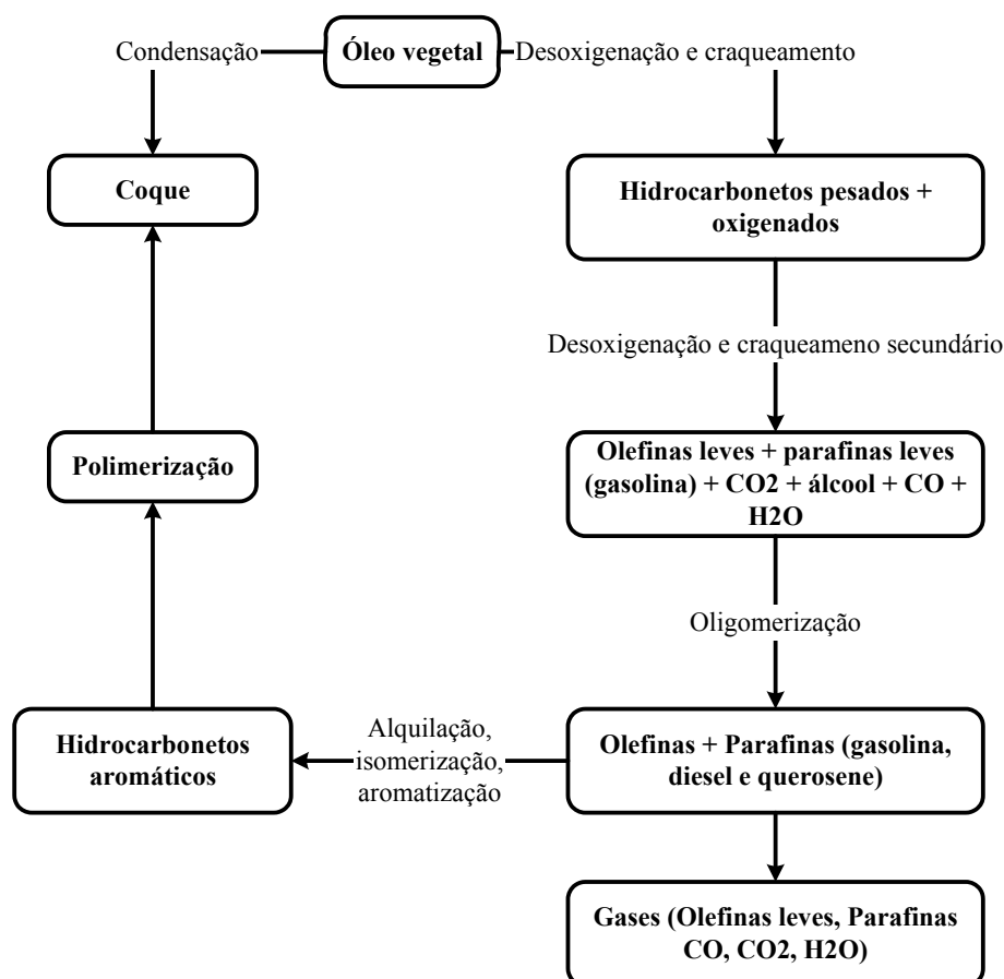
Figura 2. 1 – Rota de reação para o craqueamento de óleos vegetais.
