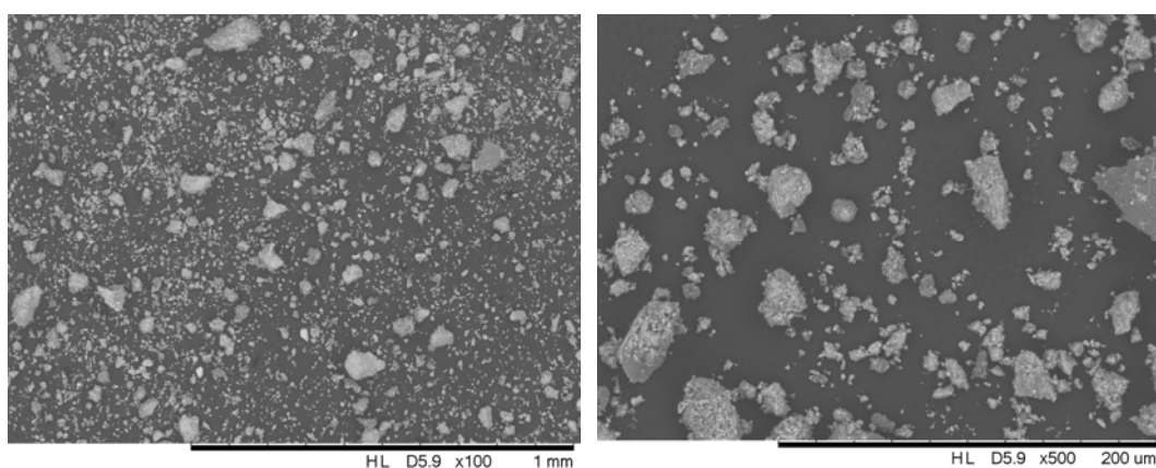
Figura 6. 11 – Microscopia eletrônica de varredura para a lama vermelha ativada quimicamente com 2M HCl.
