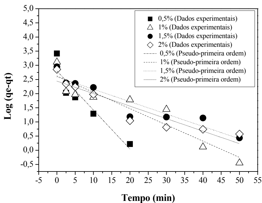
Figura D. 11 - Modelo cinético de pseudo-primeira ordem da adsorção de ácidos graxos livres em lama vermelha ativada quimicamente com 2M HCl.
