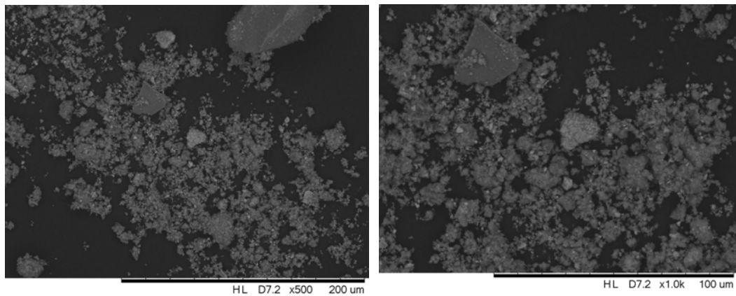
Figura 6. 8 – Microscopia eletrônica de varredura para a lama vermelha ativada termicamente a 400°C.
