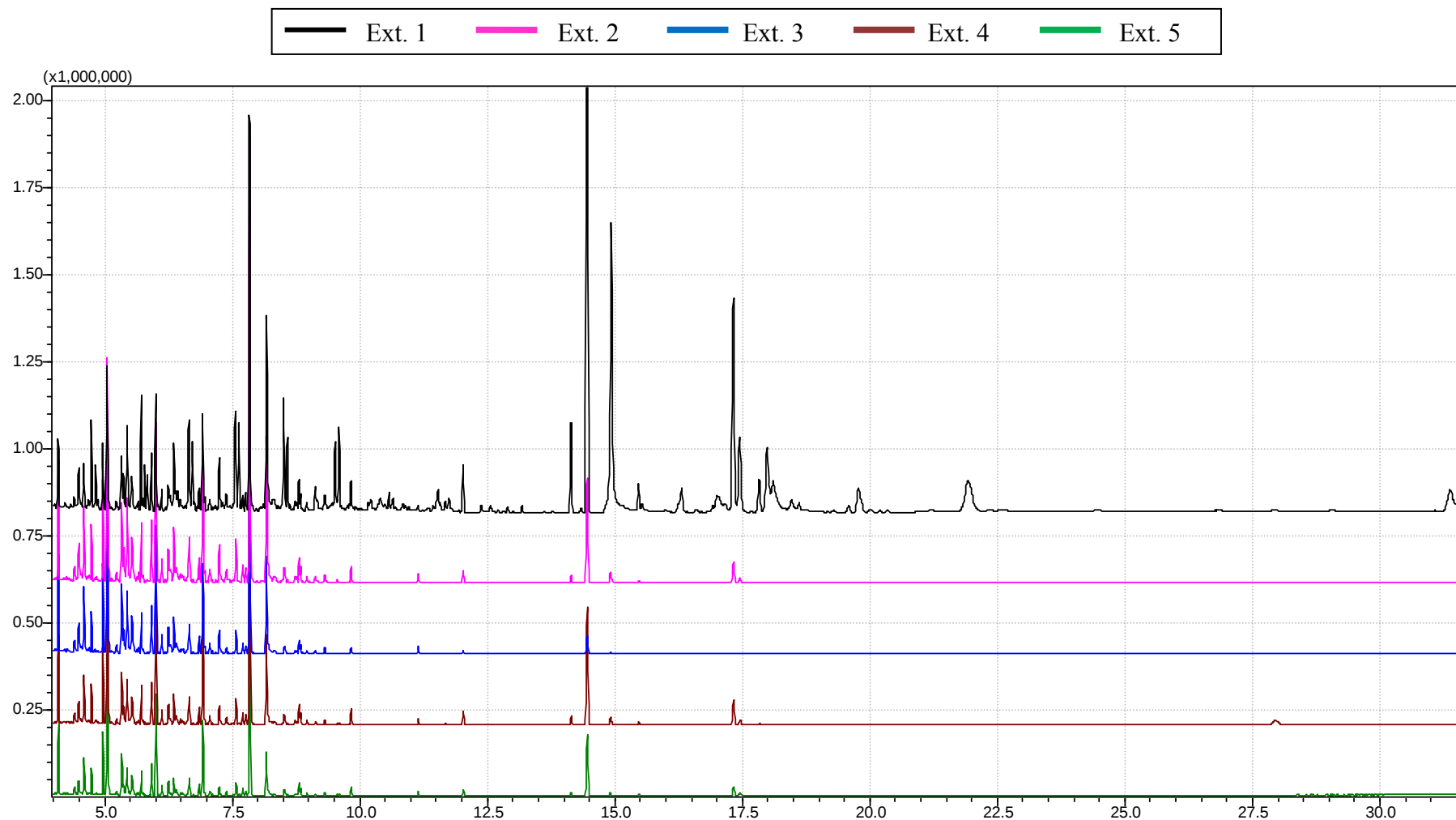
Figura C. 2 - Cromatogramas da fase extrato obtidos após a extração líquido-líquido com diferentes teores de água no solvente combinado.
