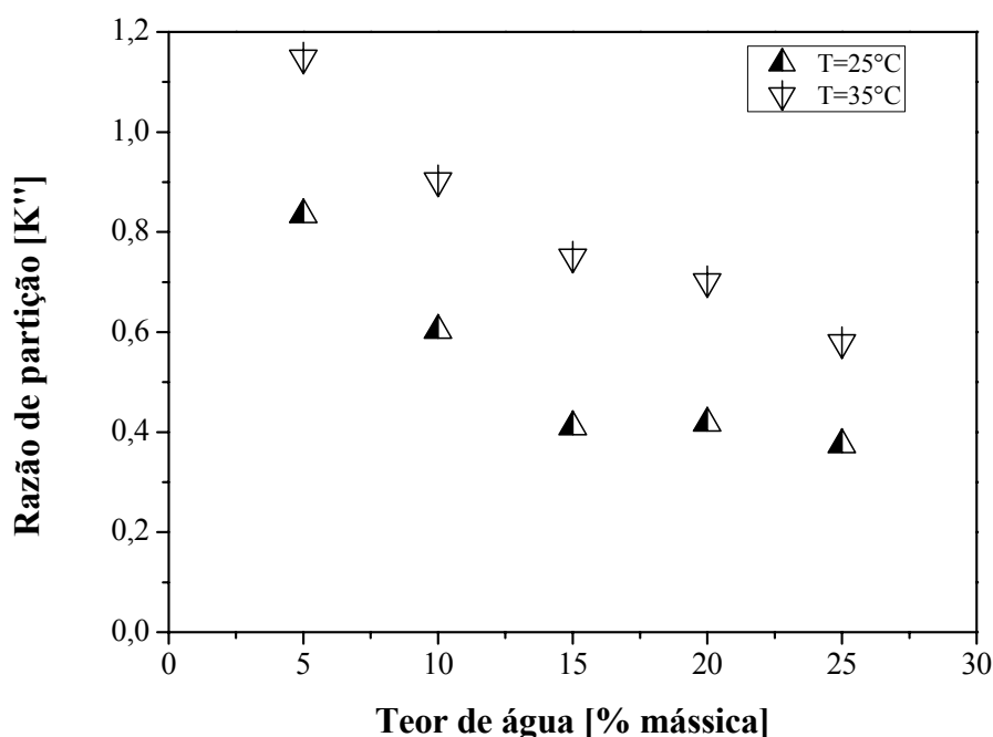
Figura 5. 6 – Razão de partição dos AGL versus teor de água para diferentes temperaturas (álcool metílico + água).
