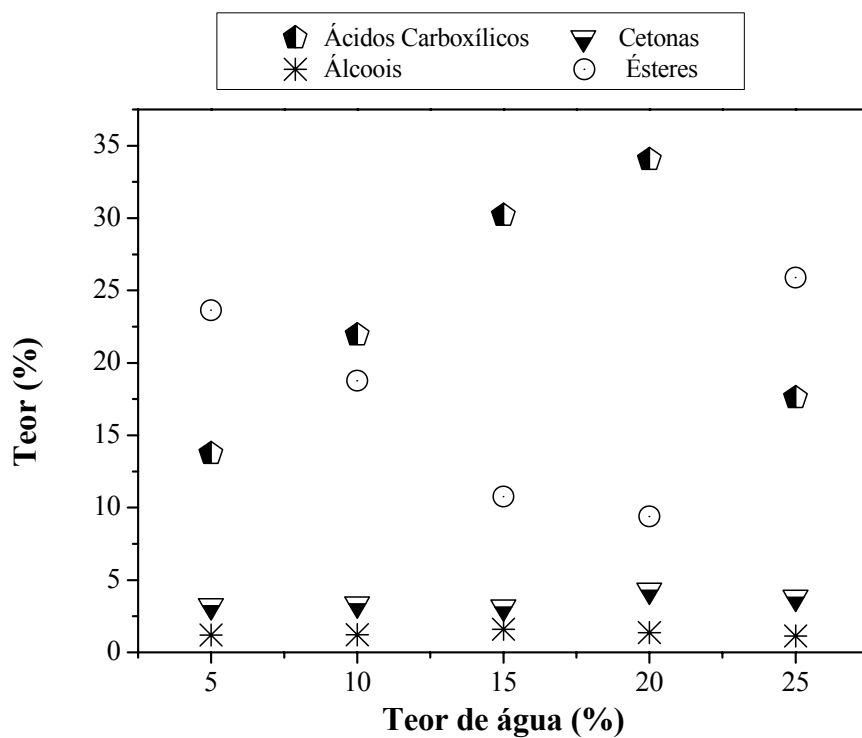
Figura 5. 15 – Efeito do teor de água no solvente combinado (álcool metílico + água) sobre a distribuição das classes de compostos oxigenados presentes nas fases refinadas.
