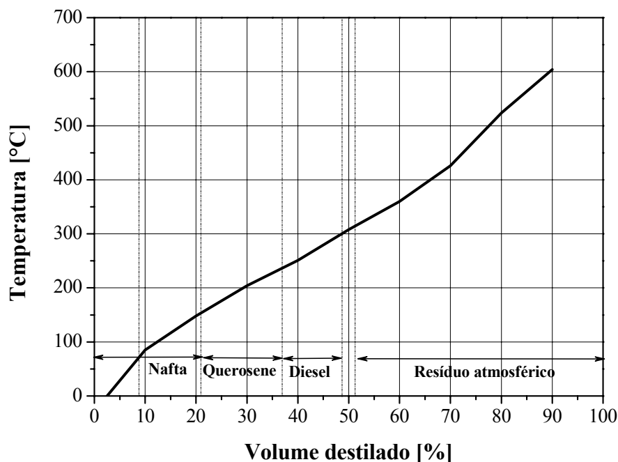
Figura 4. 1 – Curva PEV do óleo bruto na torre de destilação atmosférica.
