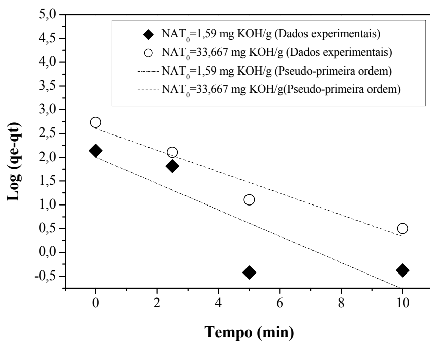
Figura D. 3 - Modelo cinético de pseudo-primeira ordem da adsorção de ácidos graxos livres em lama vermelha ativada termicamente a 400°C.
