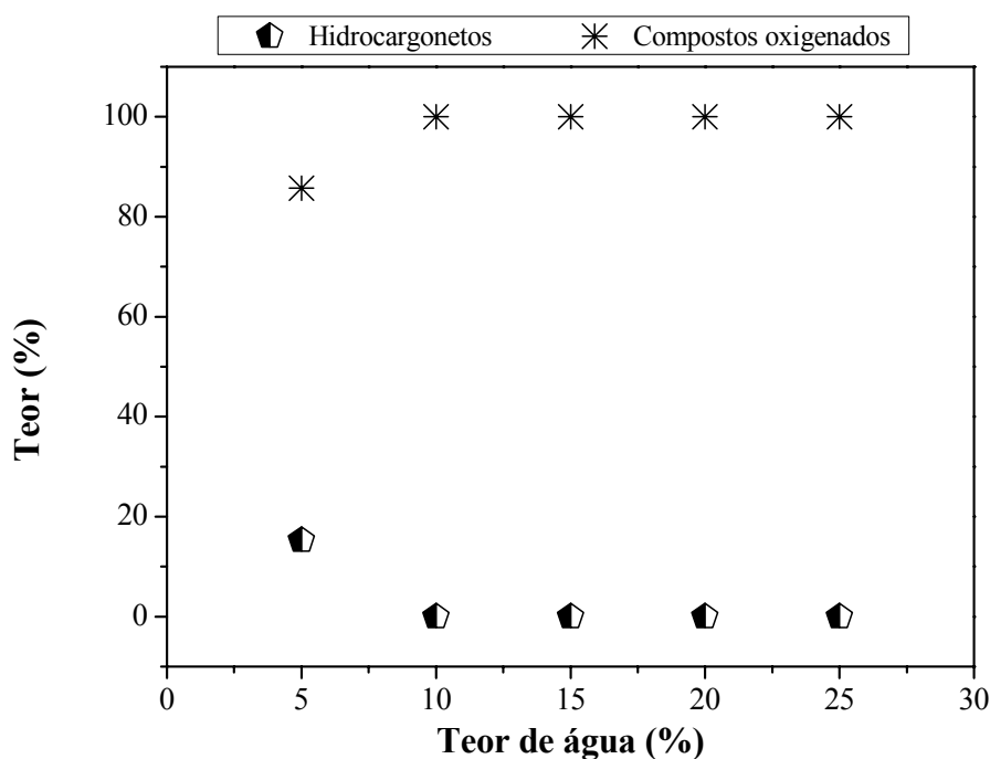
Figura 5. 14 – Efeito do teor de água no solvente combinado (álcool metílico + água) sobre a concentração de hidrocarbonetos e compostos oxigenados presentes nas fases extratos.
