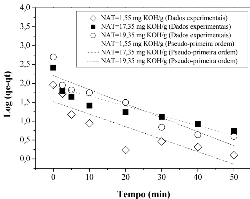
Figura D. 1 - Modelo cinético de pseudo-primeira ordem da adsorção de ácidos graxos livres em alumina ativada a 450°C.
