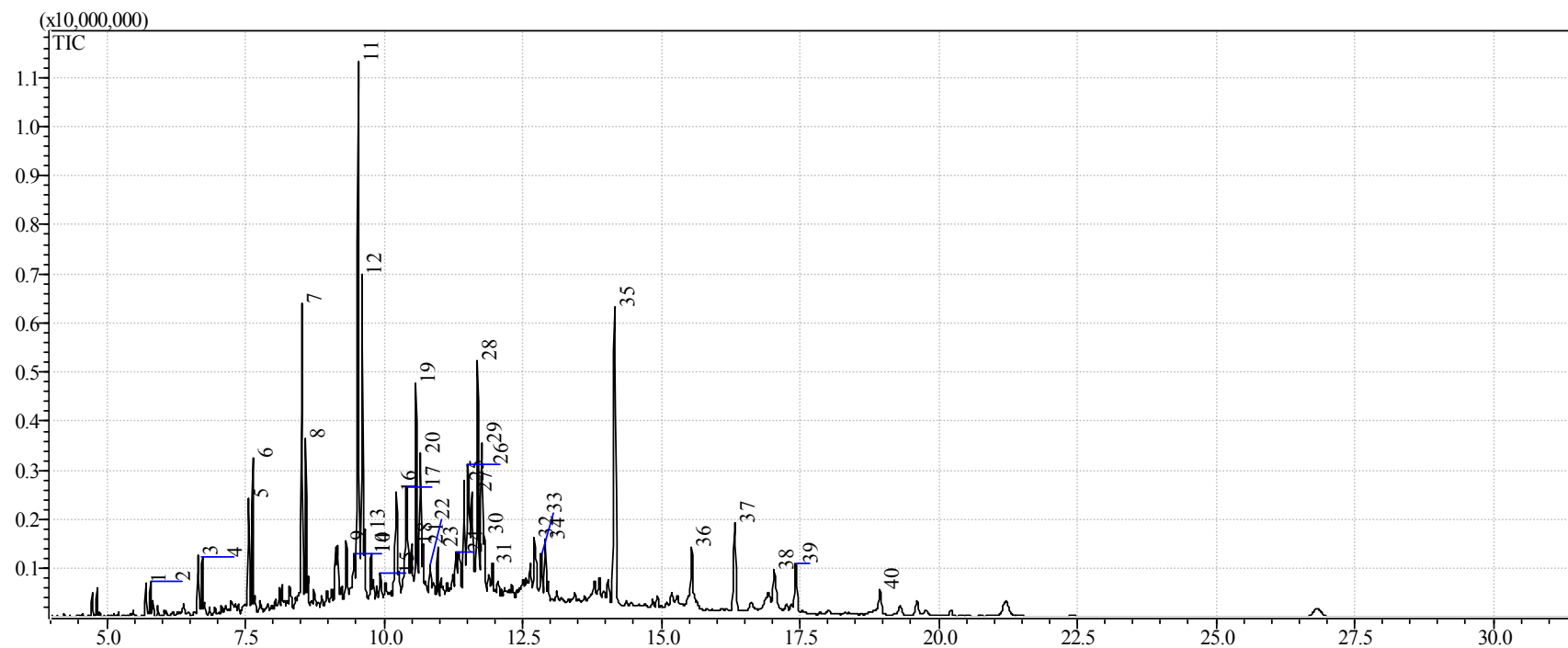
Figura B. 4 - Cromatograma da fração destilada na faixa de diesel pesado (305-400°C) oriunda do fracionamento do PLO (20% de carbonato de sódio).
