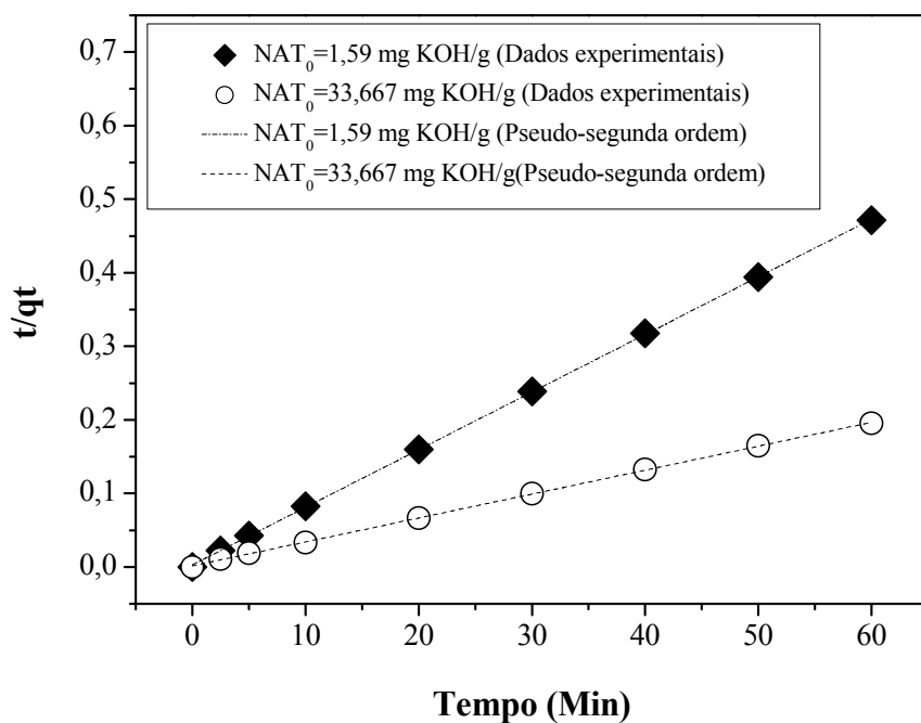
Figura D. 6 - Modelo cinético de pseudo-segunda ordem da adsorção de ácidos graxos livres em lama vermelha ativada termicamente a 600°C.
