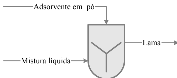
Figura 6. 1 – Adsorção em batelada em tanque agitado.
