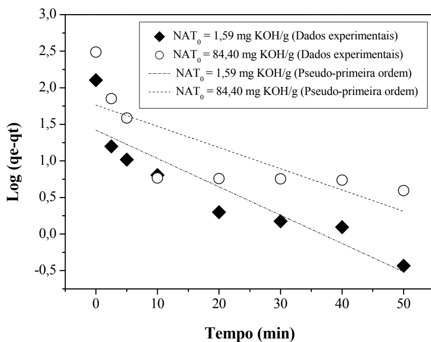
Figura D. 5 - Modelo cinético de pseudo-primeira ordem da adsorção de ácidos graxos livres em lama vermelha ativada termicamente a 600°C.
