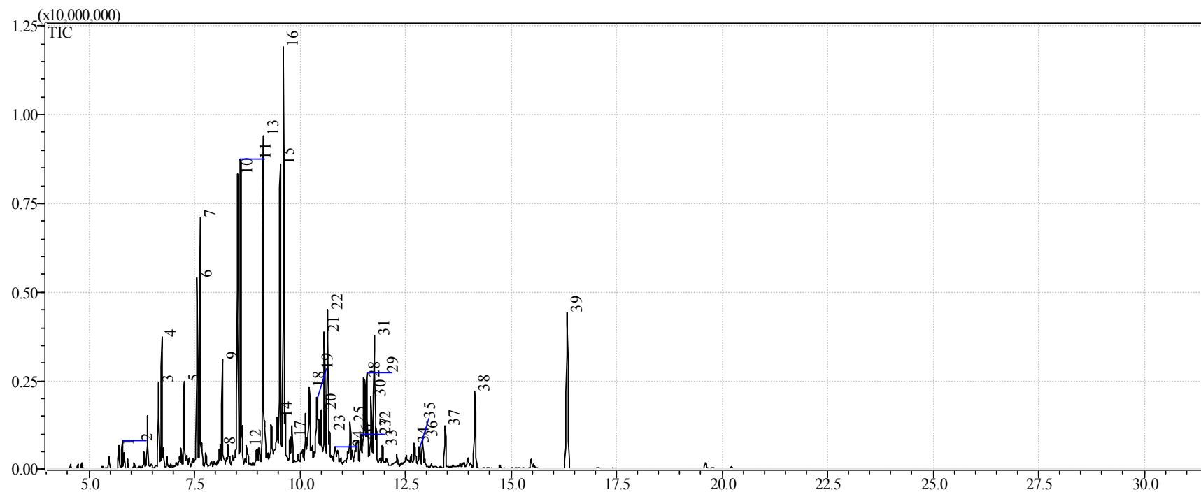
Figura B. 1 - Cromatograma da fração destilada na faixa de diesel pesado (305-400°C) oriunda do fracionamento do PLO (5% de carbonato de sódio).
